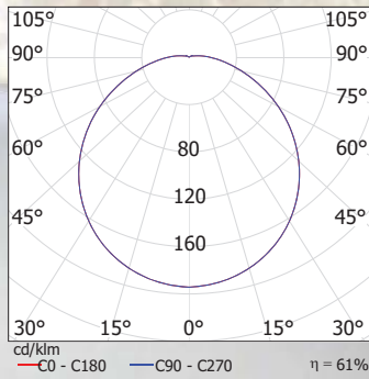
SI Diffuser
