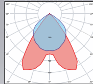
cd/klm \eta = 64\% — C0 - C180 — C90 - C270
